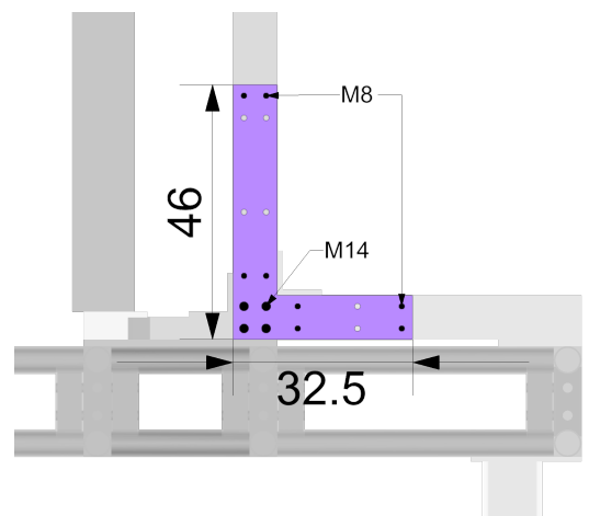
L-Platte Stahl, Maßstab 1:15
