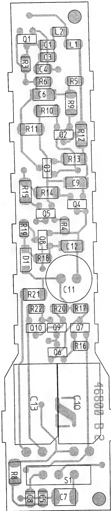
K 6 P, GEDRUCKTE SCHALTUNG, BESTÜCKUNGSSEITE K 6 P, PRINTED CIRCUIT BOARD, COMPONENT SIDE
